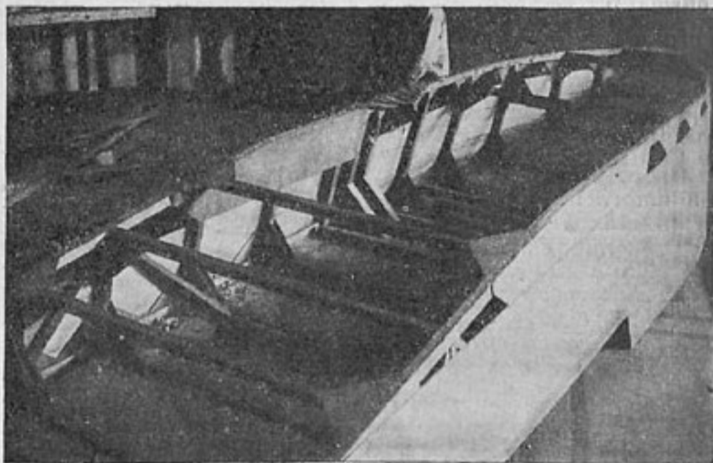
Строящийся глиссер Вхутейна
