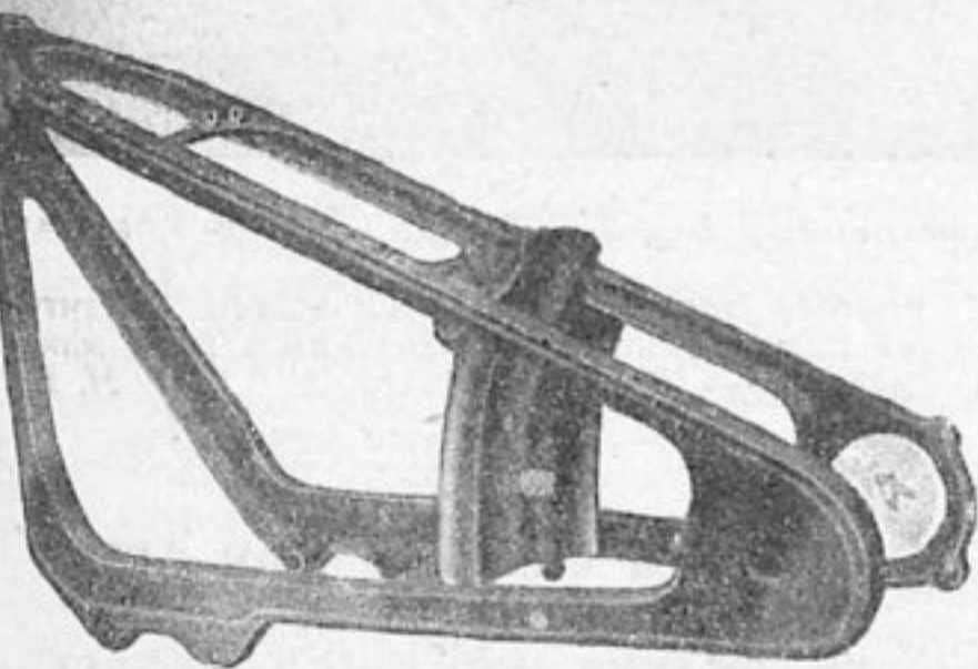
Прессованная рама „Цюндапп“
